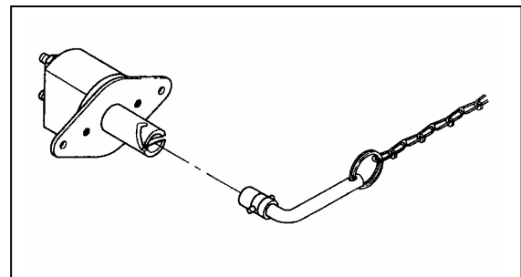
Afb. 18 Hoofdschakelaar
