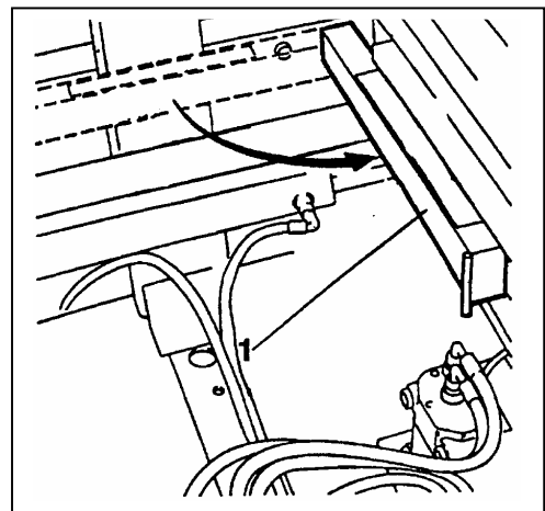
Afb. 25 Veiligheidsteun
