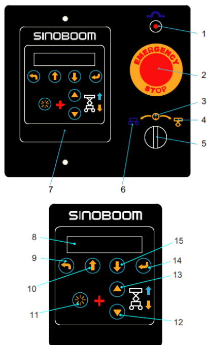
Afbeelding 6-1 Grondbediening
