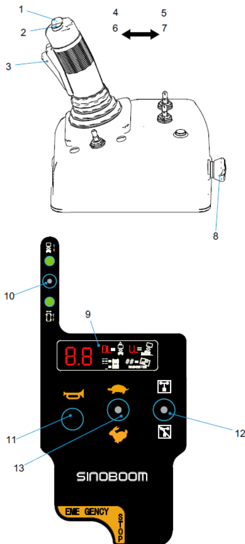
Afbeelding 6-2 platformbediening (SINOBOOM)
