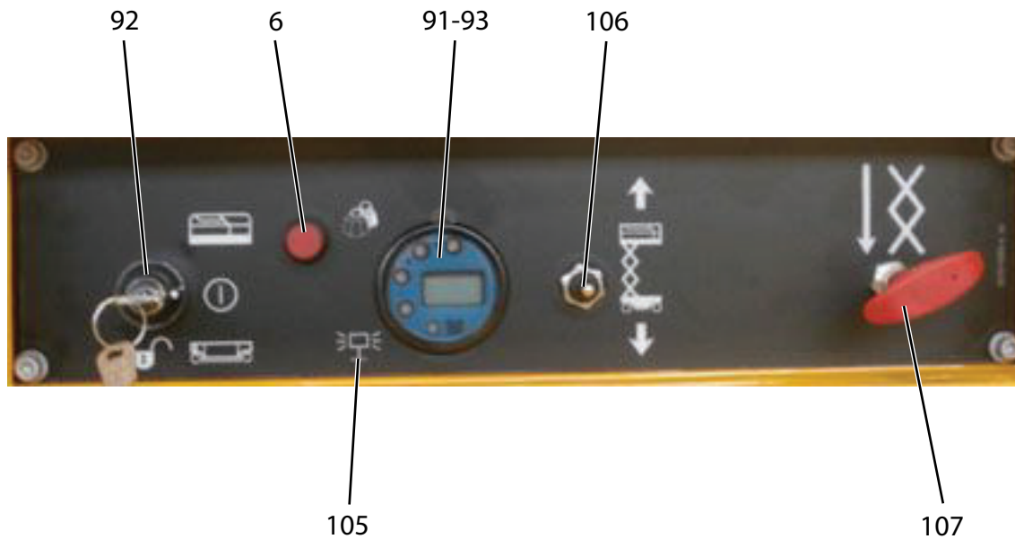
Noodstopdrukknop
