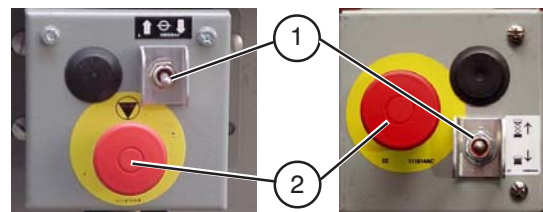
Figuur 2-3. Basisbedieningspost
