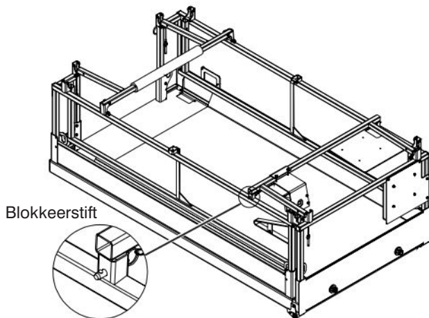
Figuur 2-12b. Alle relingen toegevouwen
