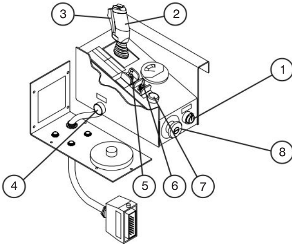
Figuur 2-10. Bedieningspaneel
