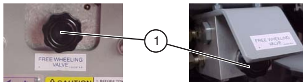
Figuur 2-20. Vrijloopklep
