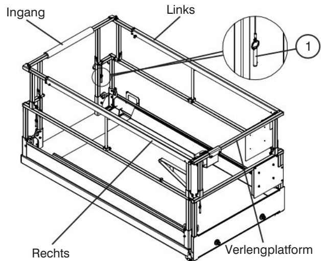
Figuur 2-12a. Opvouwbaar relingsysteem
