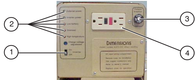
Figuur 2-15. 1500 W gelijkstroomomvormer
