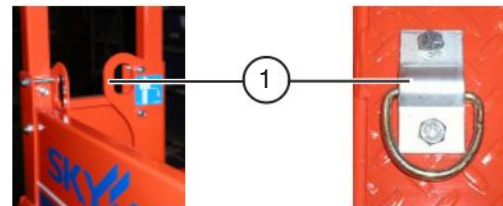
Figuur 2-13. Lijnaanhechtingsring
