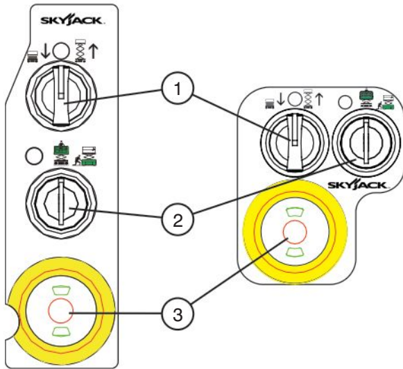
Figuur 2-2. Basisbedieningsconsole
