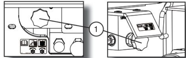
Figuur 2-7. Vrijloopklep
