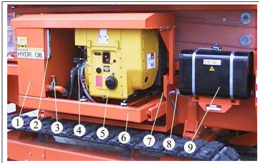
Afb. 15 Dieselmotor
