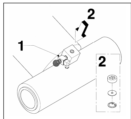
Afb. 10 Leiding-/slangbreukbeveiliging
