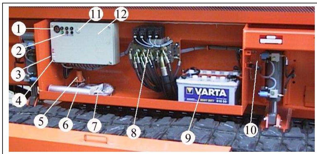
Afb. 16 Ventiellkast
