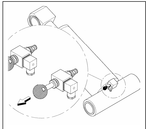
Afb. 9 Nooddaalvoorziening
